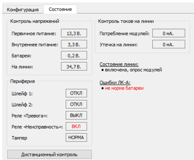
Рис. 23 Панель мониторинга состояния ЛК-А
