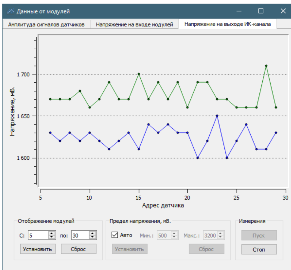
Рис. 27 Форма мониторинга напряжения на выходе ИК-канала
