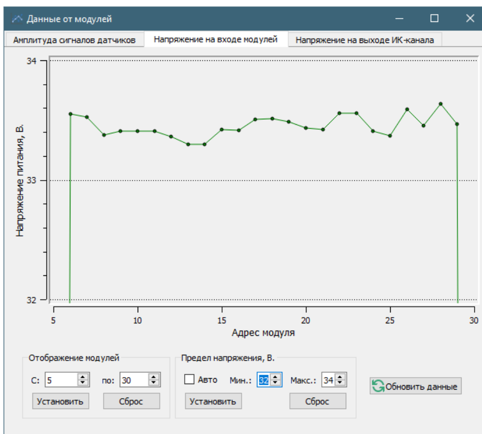
Рис. 26 Форма мониторинга напряжения на входе модуля
