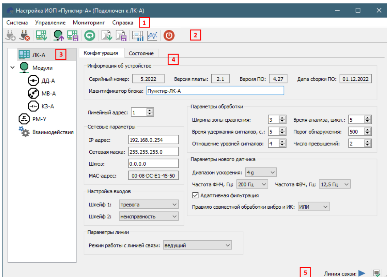
Рис. 6 Главное окно программы настройки
